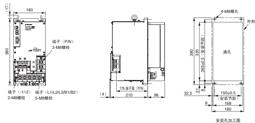
安装孔加工图
