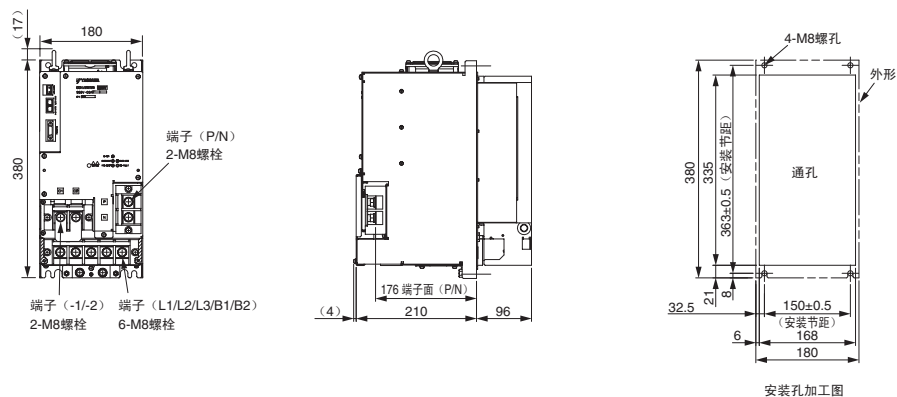
安装孔加工图
