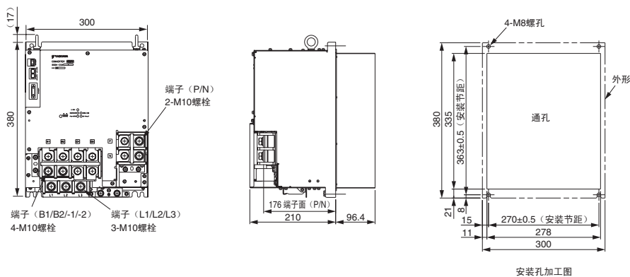
安装孔加工图
